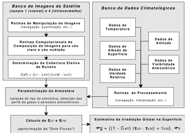
Figura 1. Diagrama em blocos do Modelo BRASIL-SR apresentando o gerenciamento e manipulação do banco de dados climatológicos e de imagens do satélite GOES-8 utilizados para alimentação do modelo.
