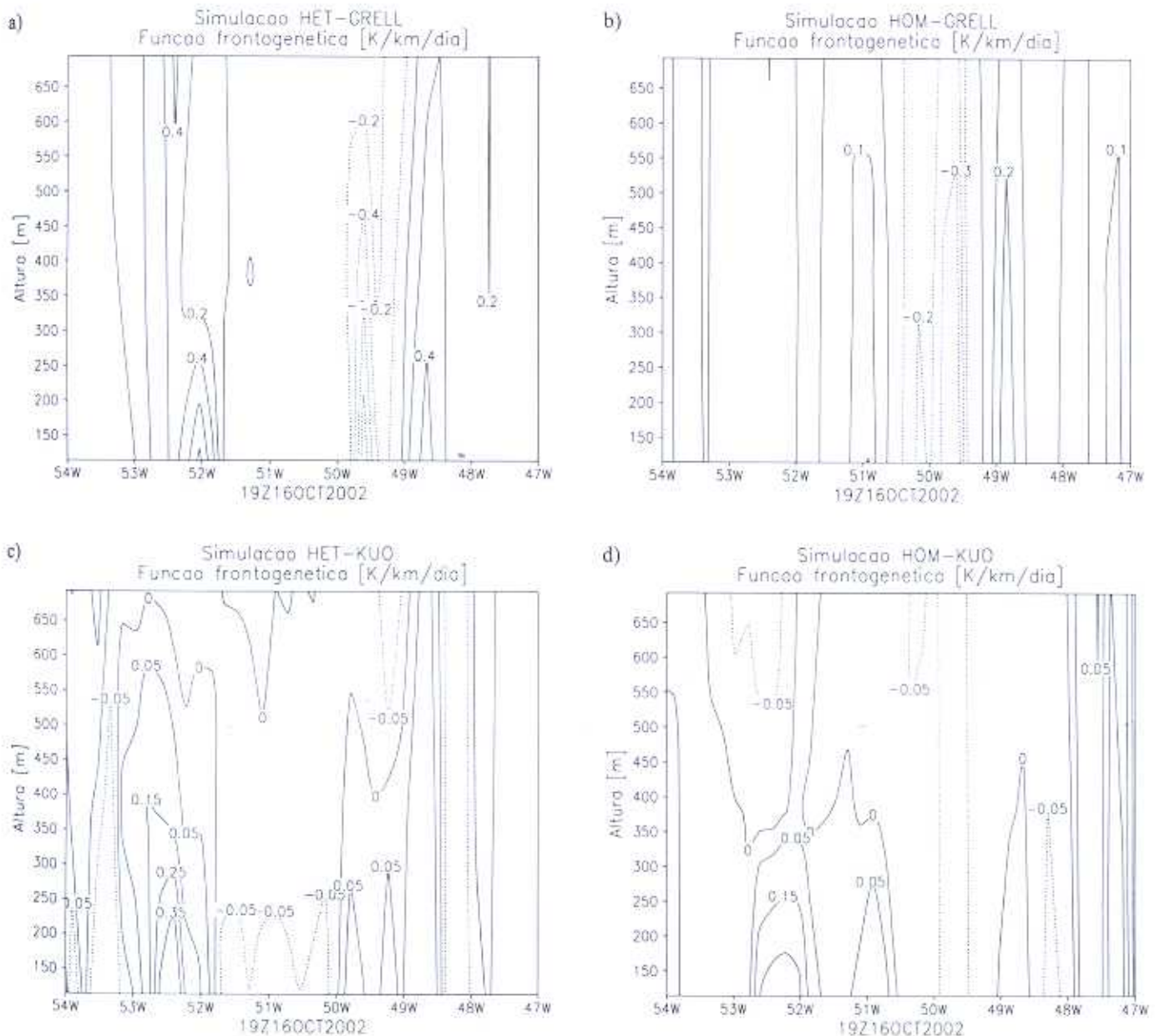
Figura 10 – Perfil vertical em 15°S da função frontogenética nos quatro experimentos principais (K/km/dia) às 19:00 UTC do dia 16 de outubro de 2002.
