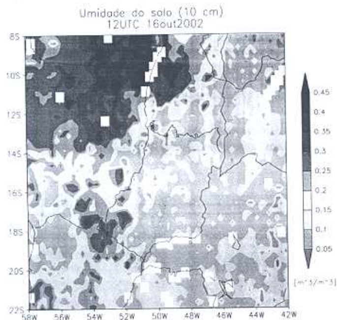
Figura 6 – Umidade do solo em Goiás às 12:00 UTC do dia 16 de outubro de 2002 ( m^3/m^3 ), obtida com a técnica de Gevaerd e Freitas (2005).
