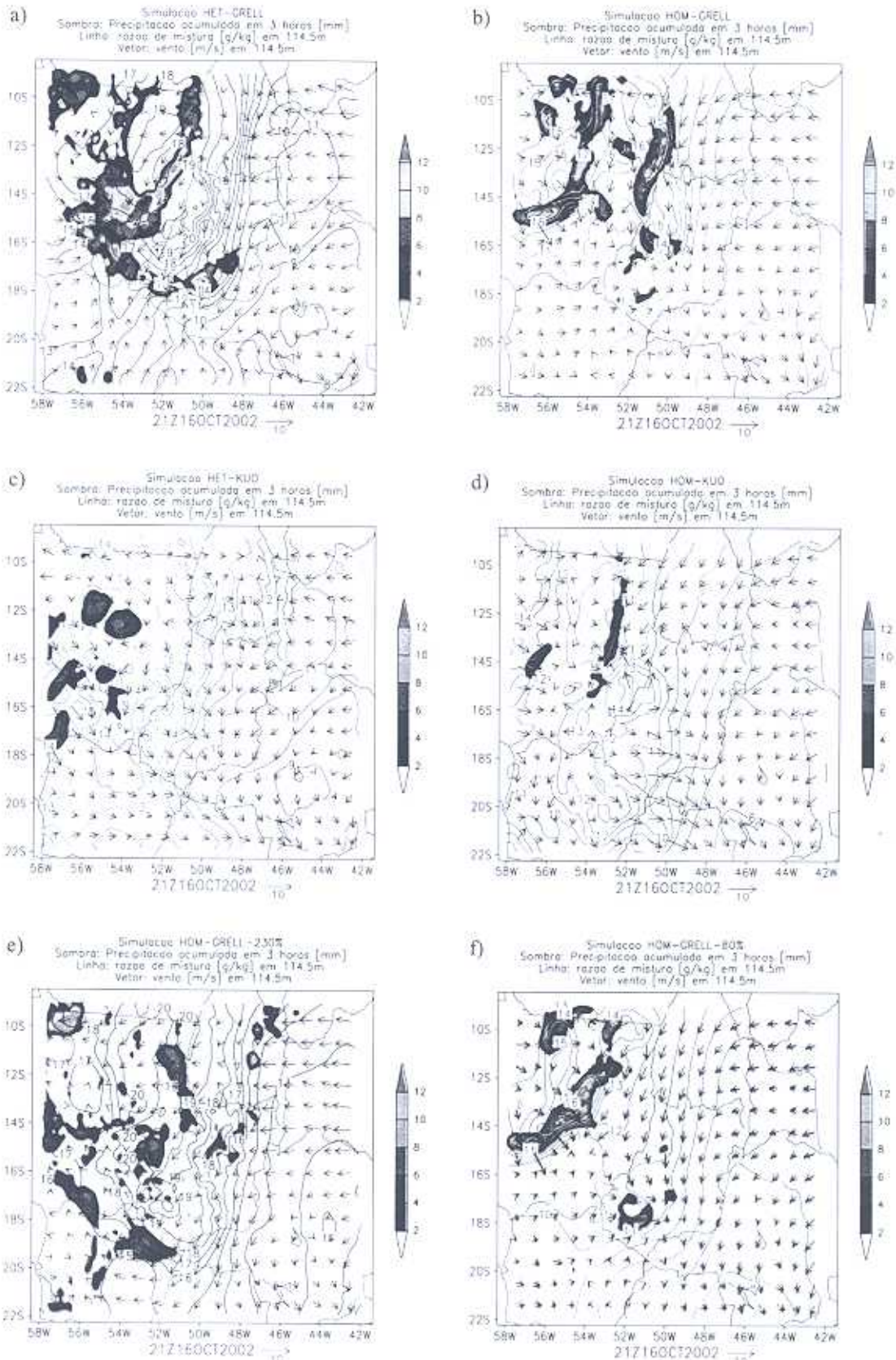
Figura 7 – Precipitação acumulada em 3 hora (mm), razão de mistura (g/kg) e vento em 114.5 m para os experimentos na grade 2, às 21:00 UTC do dia 16 de outubro de 2002.
