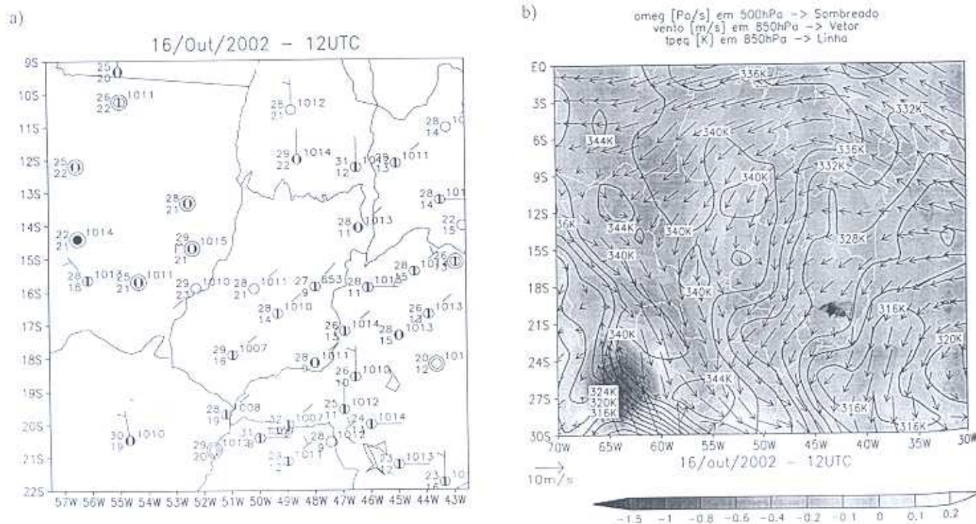
Figura 3 Dados do SYNOP para o dia 16 de outubro de 2002, às 12:00 UTC (a) e campos de velocidade vertical em 500 hPa (sombreado), vento (vetor) e temperatura potencial equivalente (linha) em 850 hPa na mesma data (b). Fonte: CPTEC/INPE.
