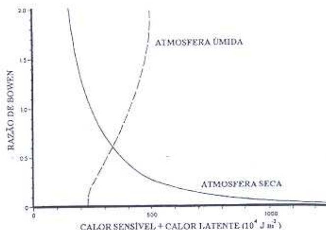
Figura 1 – Calor sensível e latente requeridos pela atmosfera para formação de nuvens convectivas versus razão de Bowen da superfície para dois perfis atmosféricos distintos (Adaptado de Rabin, 1977).
