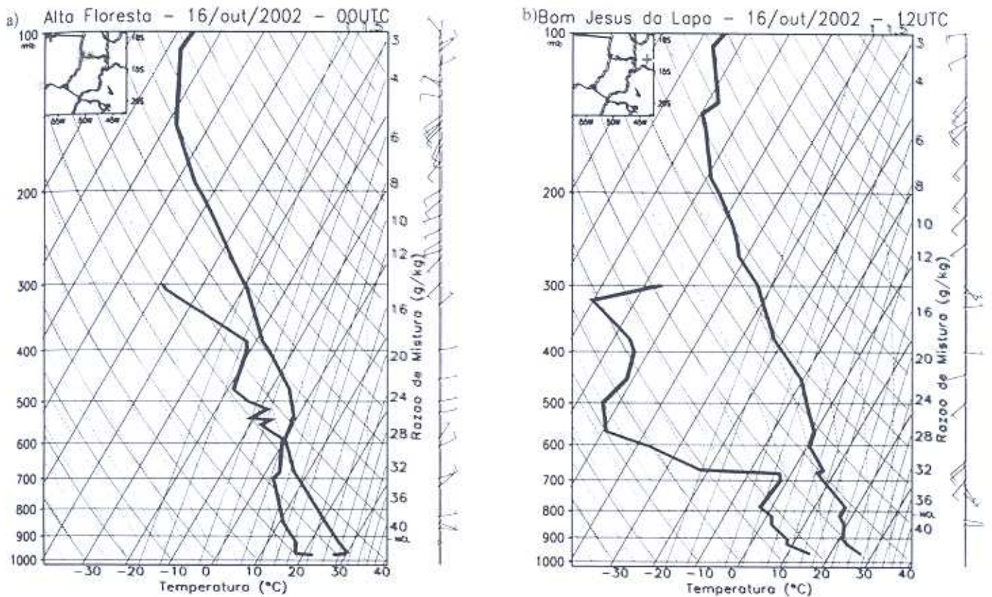
Figura 4 – Diagramas skew-T log-P para as localidades de Alto Floresta (a) e Bom Jesus da Lapa (b). Em destaque a localização destas cidades. Fonte: Laboratório Master.
