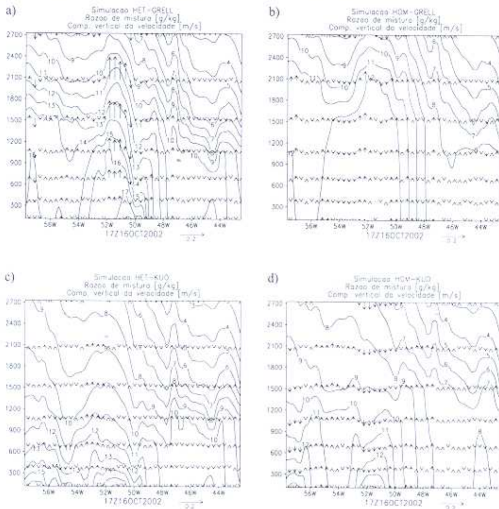
Figura 8 – Perfil vertical em 15°S da razão de mistura (g/kg) e componente vertical do vento (m/s) para as quatro simulações principais na grade 2, às 17:00 UTC do dia 16 de outubro de 2002.
