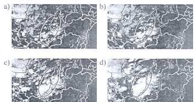
Figura 2 - Imagens de satélite GOES-8 ilustrando a propagação da linha às 17:45 (a), 18:45 (b), 20:45 (c) e 22:15 UTC (d), do dia 16 de outubro de 2002. Fonte: CPTEC/INPE.
