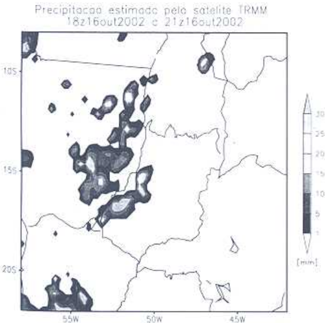
Figura 5 – Estimativa de precipitação (mm) acumulada entre 18:00 e 21:00 UTC do dia 16 de outubro de 2002, período que explica a maior parte da precipitação associada ao sistema. Fonte: TRMM.
