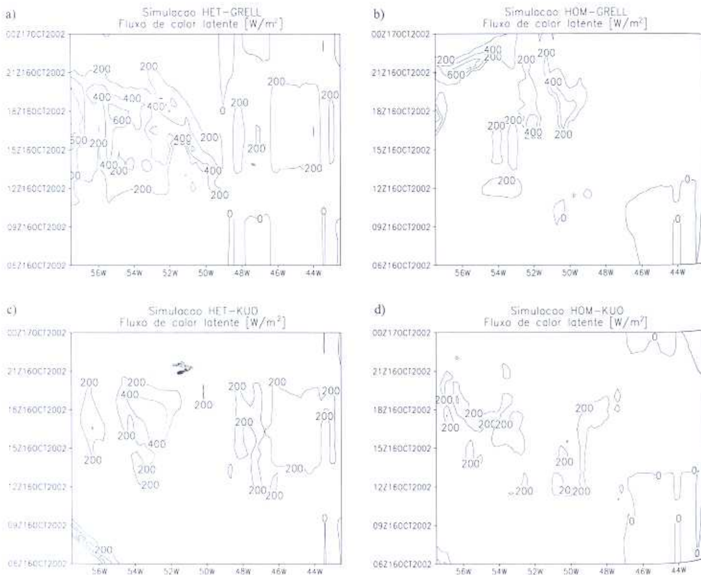
Figura 9 – Série temporal em 15°S do fluxo de calor latente nos quatro experimentos principais ( W/m^2 ), a partir de 06:00 UTC do dia 16 de outubro de 2002
