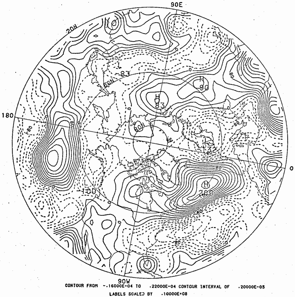
Fig. 4.5 - Configuração média de desvios de vorticidade relativa (200mb), em projeção estereográfica polar, para anos de alta pluviosidade no Nordeste (dezembro de 1963, dezembro de 1972 e janeiro de 1974).
