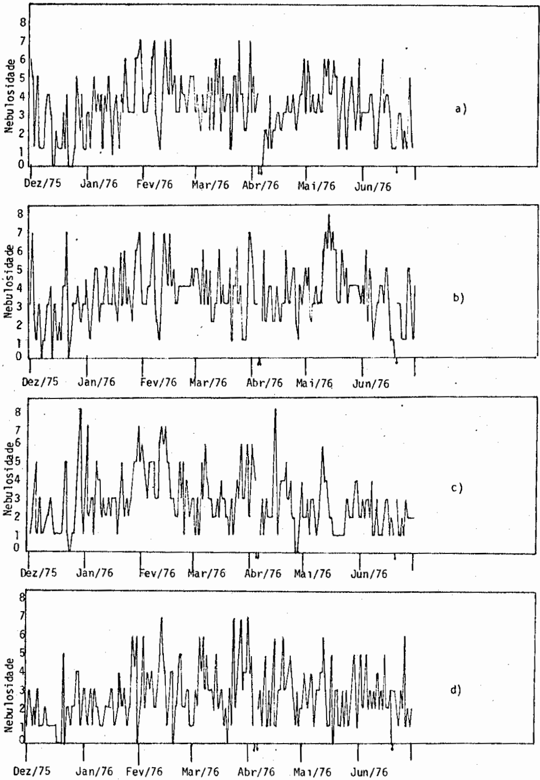
Fig. 3.16 - Séries nebulosidade versus tempo, dezembro/1975 a junho/1976, para os seguintes quadrados de Marsden: a) 005 1; b) 004 2; c) 304 1; e d) 303 2.
