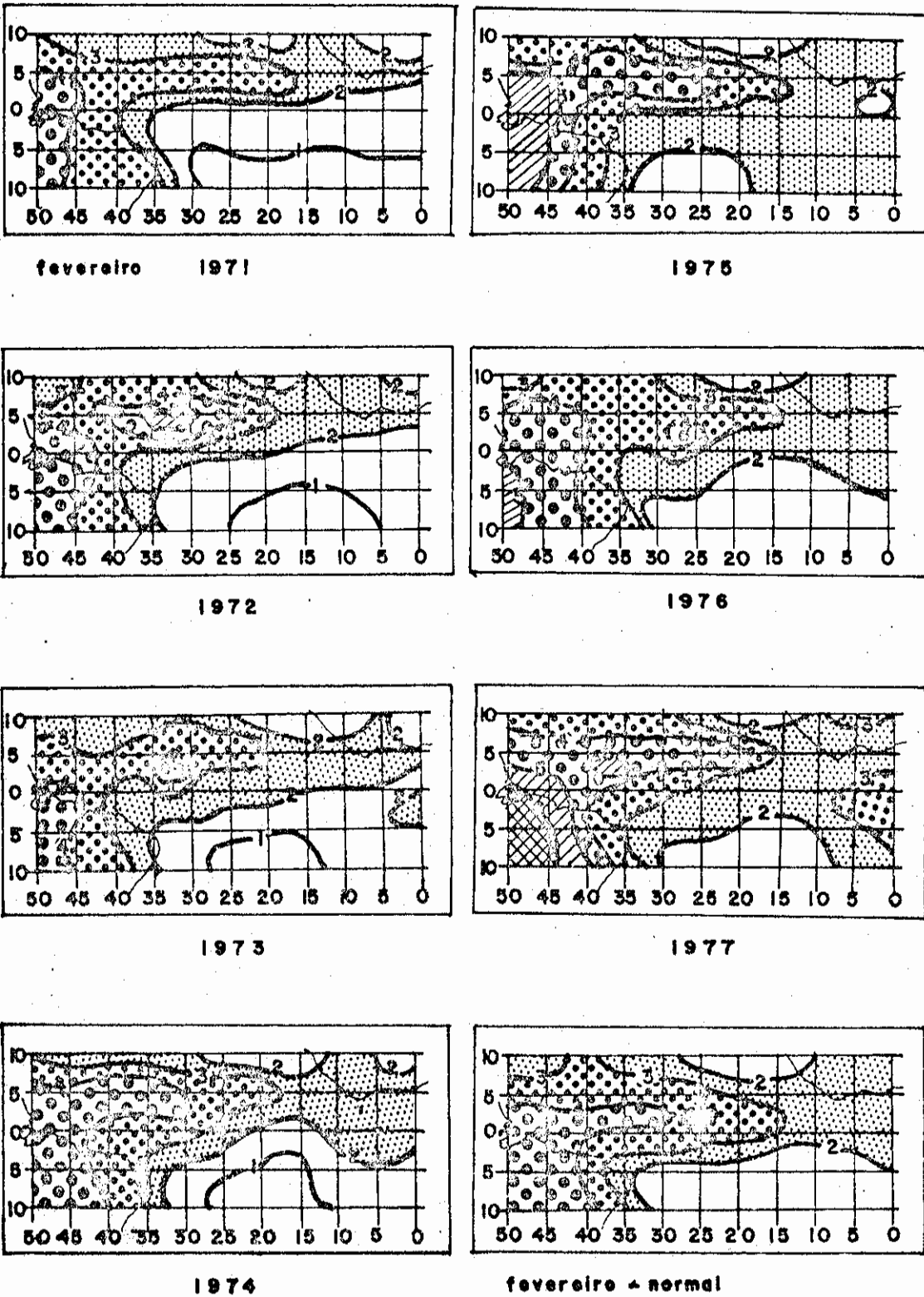
Fig. 3.5 - Cartas de brilho mēdio mensal e normal do mēs de fevereiro, em oitavos de cēu coberto, para os anos de 1971 a 1977.
