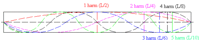
Figura 5. Comportamento dos harmônicos de um tubo com ambas as extremidades abertas.
