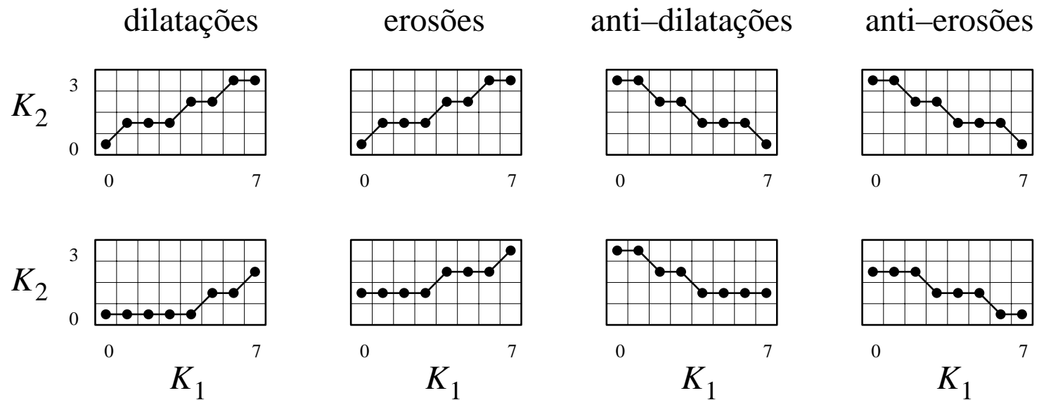
Exemplos de operadores elementares.
