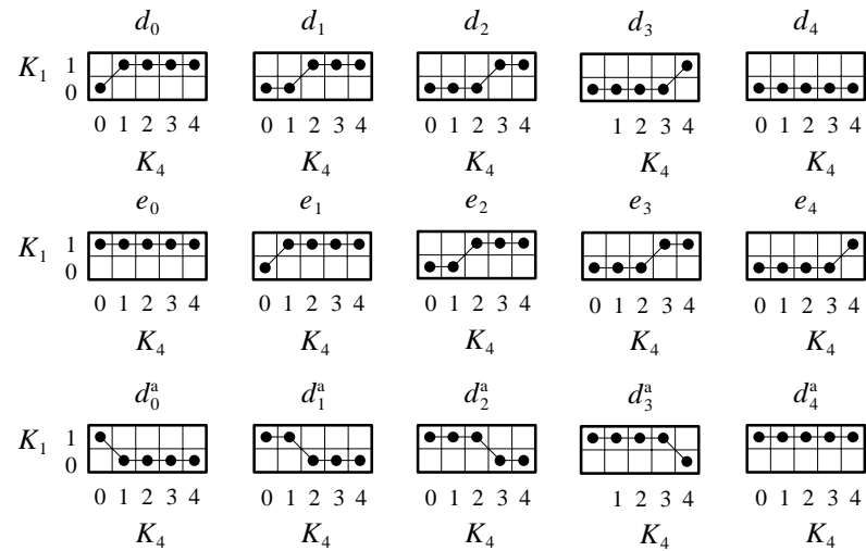
Exemplos de ELUTs para dilatação, erosão e anti-dilatação.
