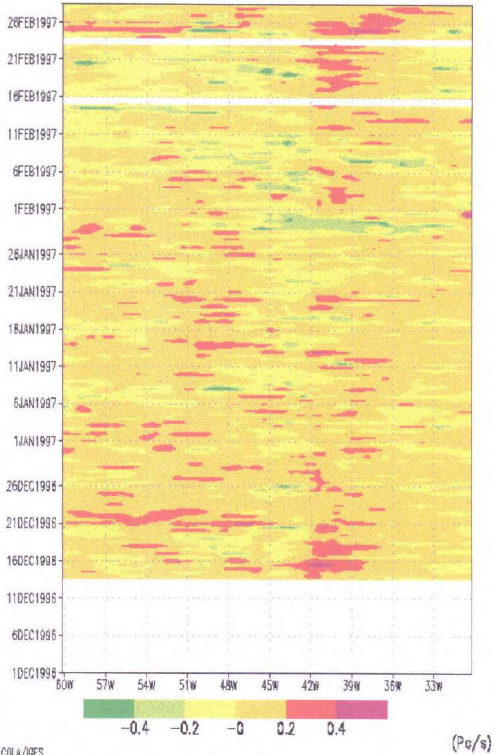
Figura 3.15: Série temporal da componente vertical do vento das previsões de 24h durante o período de dezembro de 1996, janeiro e fevereiro de 1997 (DJF) no nível de 750hPa.
