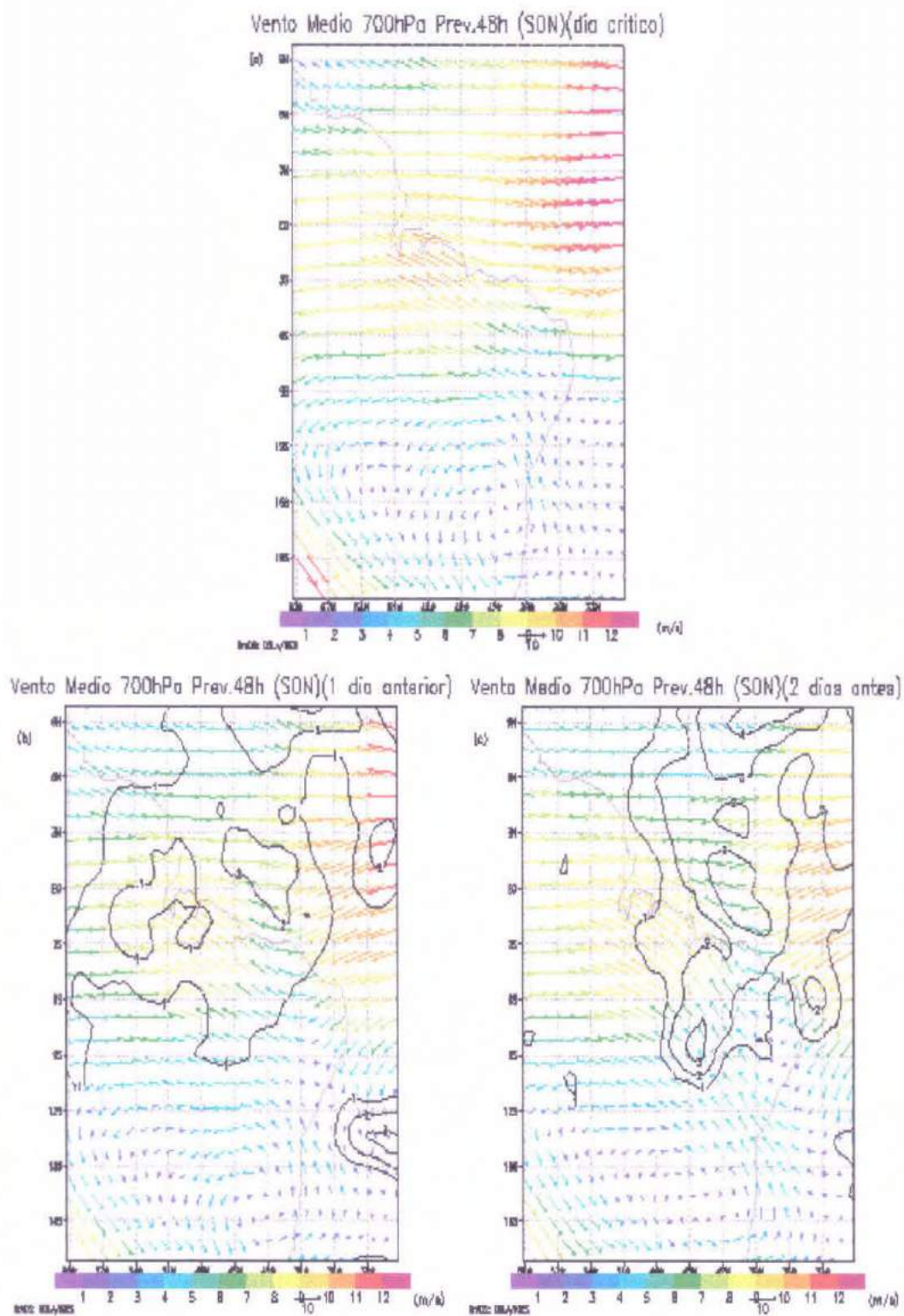
Figura 3.50: Campo médio do Nordeste dos ventos ocorridos nos dias críticos durante o período de setembro, outubro e novembro de 1997 (SON) das previsões de 48h no nível de 700hPa.
