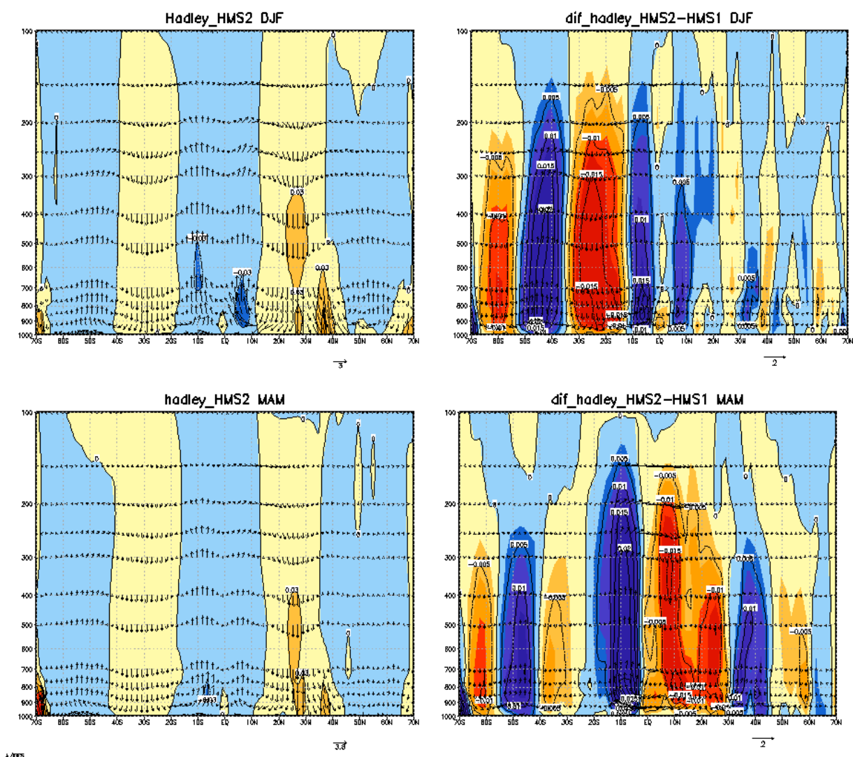
Figura 4.22 – (contorno) Velocidade vertical ( 10^2 \times \text{Pa s}^{-1} ) e o (vetor) movimento vertical ( \text{m.s}^{-1} ) na seção transversal zonal 70°S a 70°N (média entre 180°W a 180°E), para as quatro estações do ano (DJF, MAM, JJA e SON): (esquerda) HMS2 e (direita) a diferença entre os períodos. (continua)
