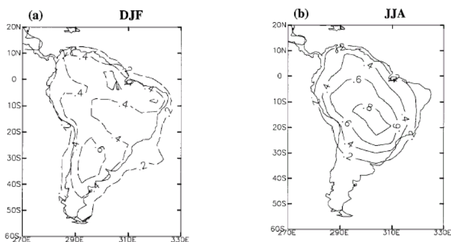
Figura 2.3 – Variação média da temperatura do ar à superfície, de 19 modelos do PMIP, entre o período do HM e CP, para (a) DJF e (b) JJA. Desvio padrão entre modelos (c) DJF e (d) JJA. As unidades são ^{\circ}\text{C} . A grade dos modelos é 5^{\circ} \times 5^{\circ} e as linhas tracejadas indicam resfriamento. (continua)
