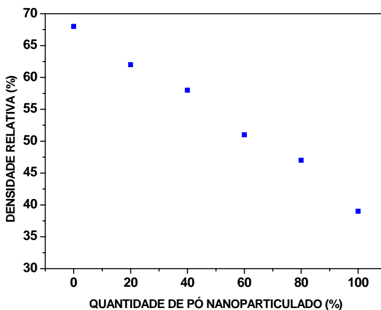
FIGURA 4.7 - Densidade relativa das cerâmicas a verde de Al_2O_3 , obtidas a partir das misturas de pós micro e nanoparticulados compactados por prensagens uniaxial e isostática.
