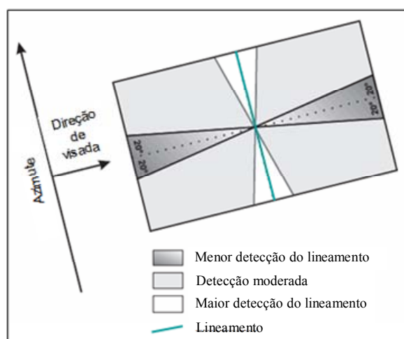
Figura 2-6 – Diagrama de supressão e realce de lineamentos de acordo com a direção de visada. Fonte: modificado de RADARSAT International (1997).
