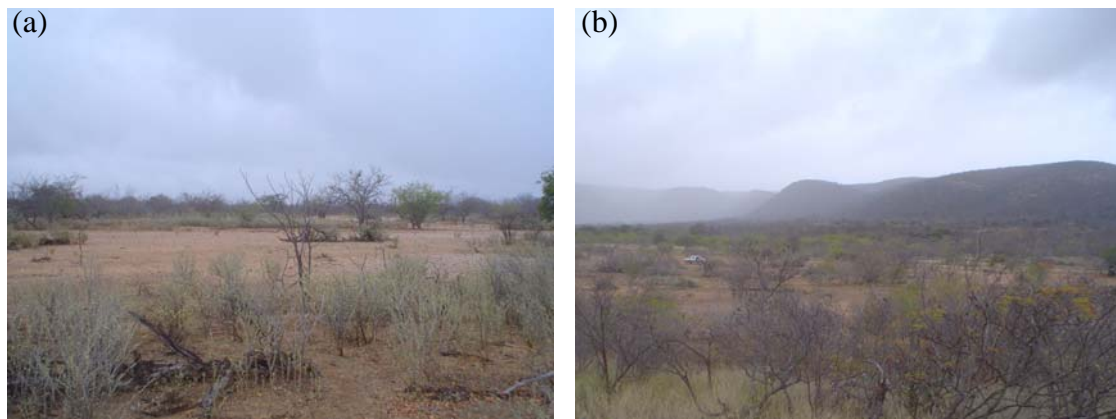
Figura 4-2 – Características geomorfológicas da área de estudo. (a) Vasta superfície de pediplanação; (b) Serra da Canabrava ao fundo.
