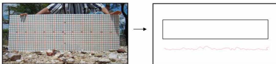
Figura 5-5 – Digitalização do perfil de rugosidade.
