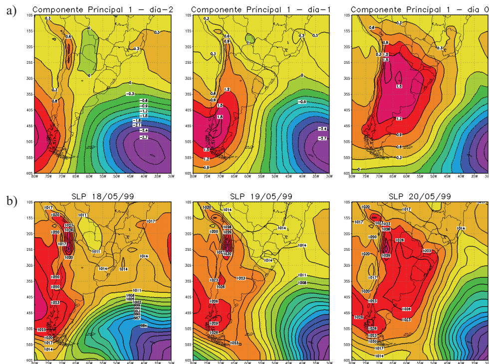
Figura 1 – (a) Primeira Seqüência de Componentes Principais (PSP1) e (b) um caso observado de pressão em superfície altamente correlacionado (8/05/99 - 20/05/99).
