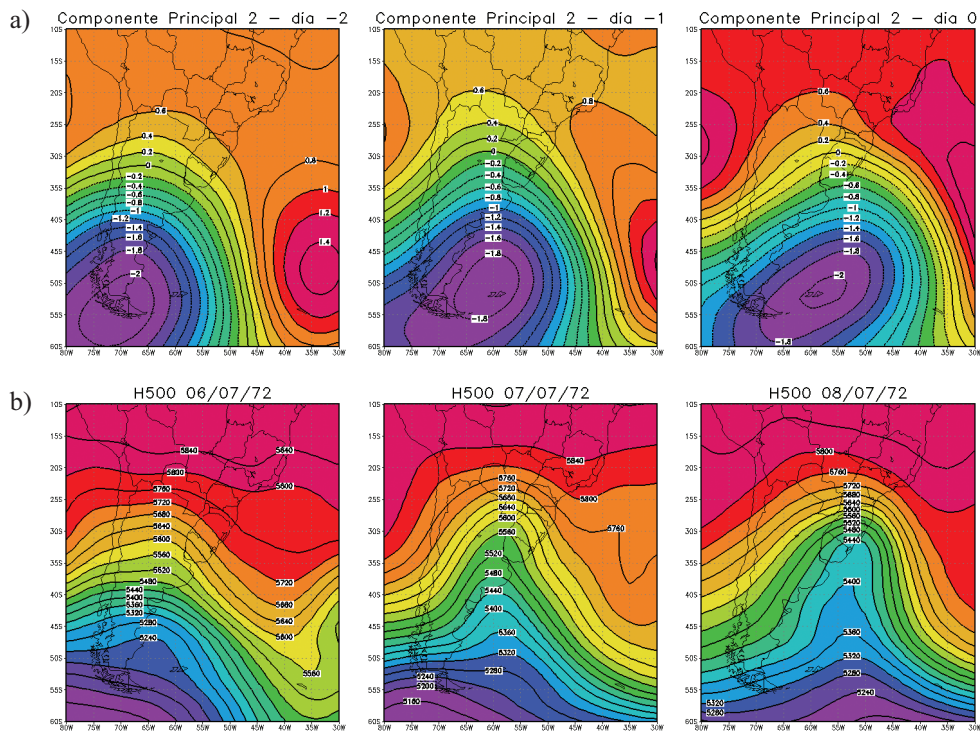
Figura 5 – (a) Segunda Seqüência de Componentes Principais (PSP 2) e (b) um caso observado de altura geopotencial em 500 hPa correlacionado (06/07/72 – 08/07/72).
