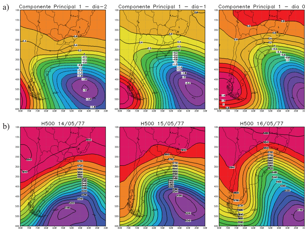
Figura 4 – (a) Primeira Sequência de Componentes Principais (PSP 1) e (b) um caso observado de altura geopotencial em 500 hPa altamente correlacionado (14/05/77 – 16/05/77).
