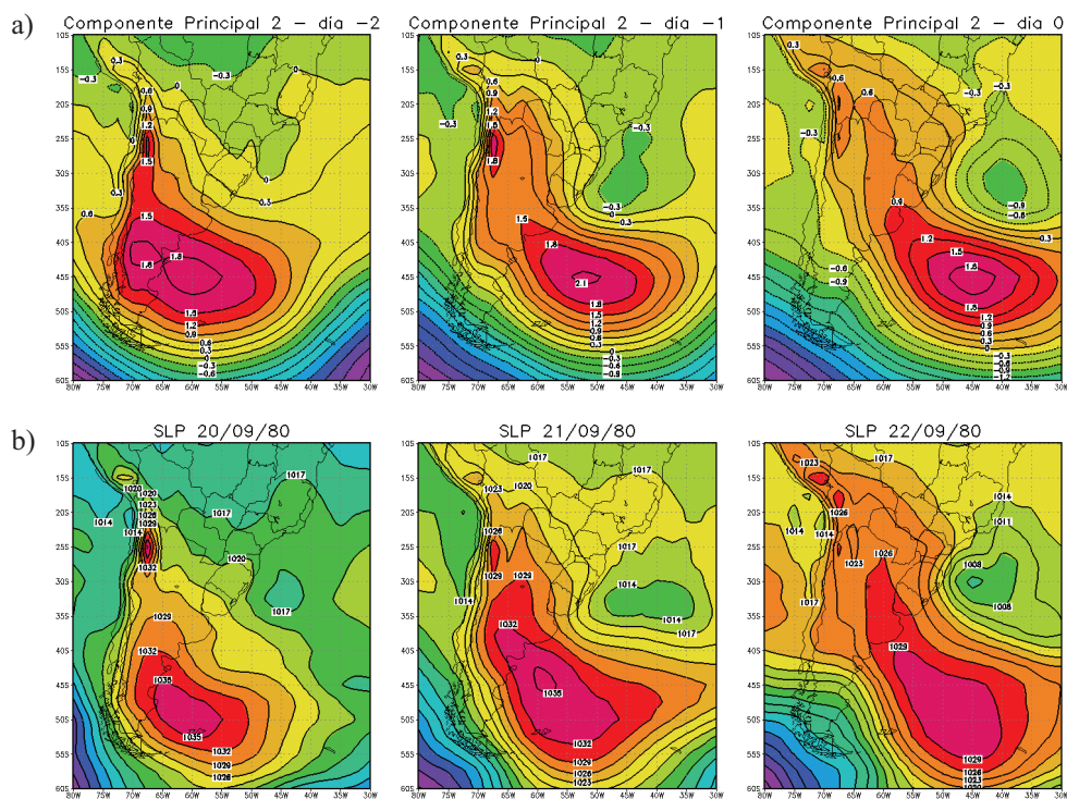
Figura 2 – (a) Segunda Sequência de Componentes Principais (PSP 2) e (b) um caso observado de pressão em superfície altamente correlacionada (20/09/80 – 22/09/80).
