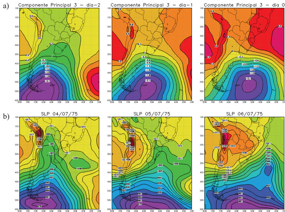
Figura 3 – (a) Terceira Seqüência de Componentes Principais (PSP 3) e (b) um caso observado de pressão em superfície altamente correlacionada (04/07/75 – 06/07/75).
