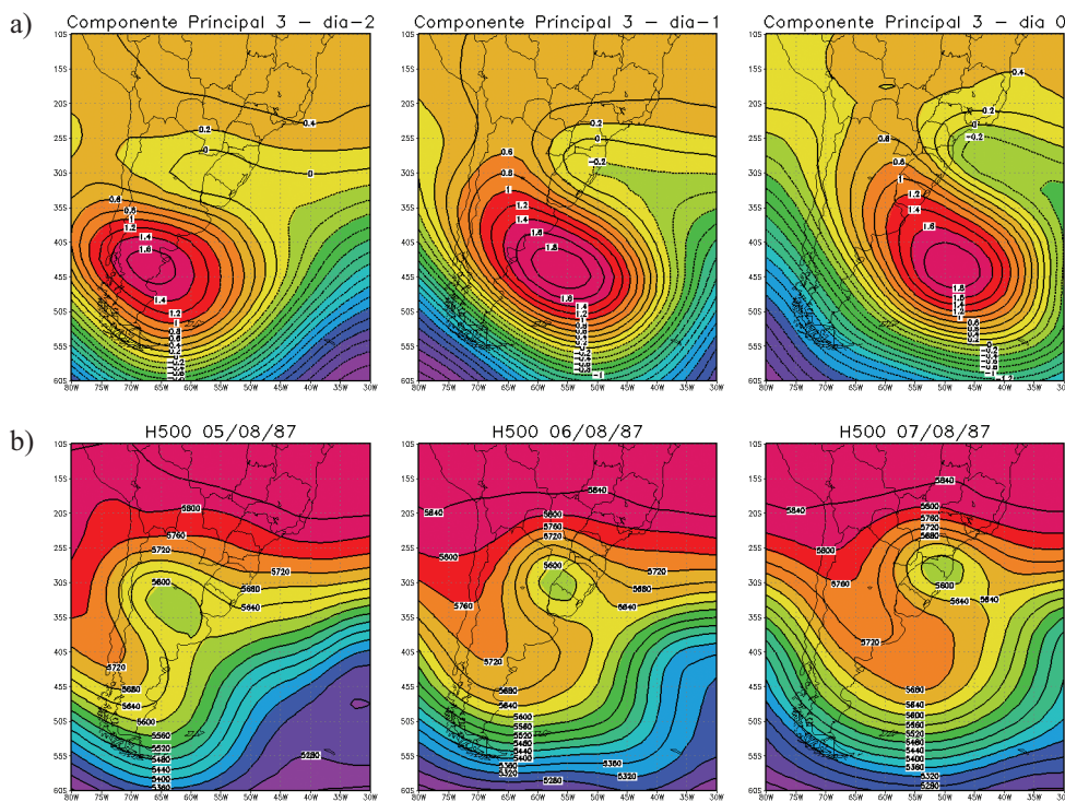
Figura 6 – (a) Terceira Seqüência de Componentes Principais (PSP 3) e (b) um caso observado de altura geopotencial em 500 hPa altamente correlacionado (05/08/87 – 07/08/87).
