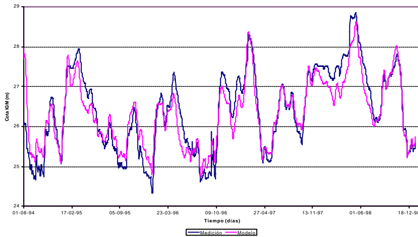
Figura 51 Comparación de niveles en la estación Esquina
