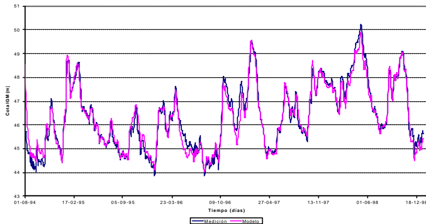
Figura 50 Comparación de niveles en la estación Corrientes
