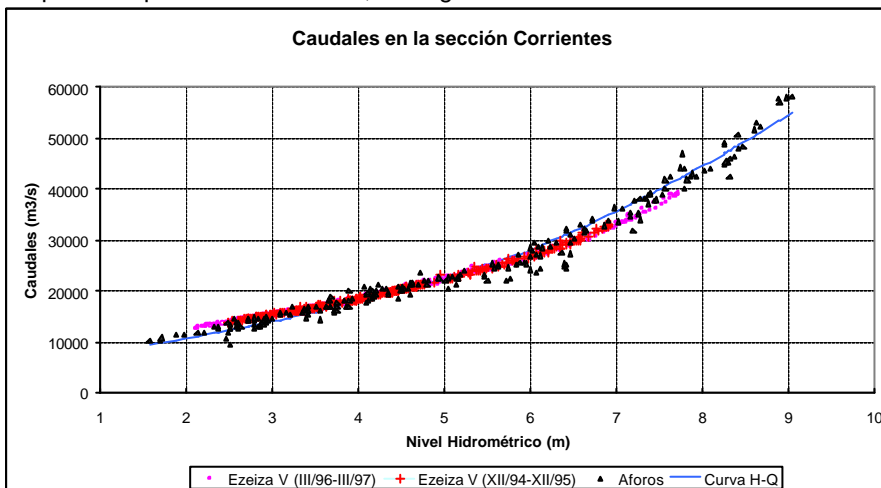
Figura 53 Comparación de caudales en la estación Corrientes
