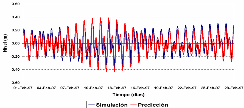
Figura 55 Comparación entre marea predicha (tablas) y calculada (modelo) en Colonia
