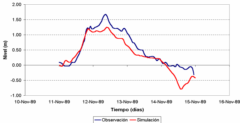
Figura 57 Comparación entre niveles registrados y calculados (Estación Torre Oyarvide)
