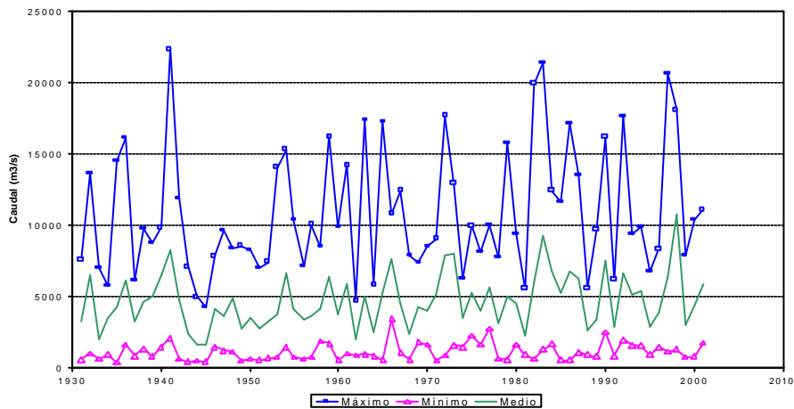
Figura 26 Máximos, mínimos y medios anuales de los caudales medios mensuales del río Uruguay en Concordia para el período 1931-2001
