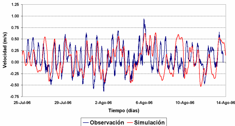
Figura 56 Comparación entre velocidades de corriente (Dirección E-O)
