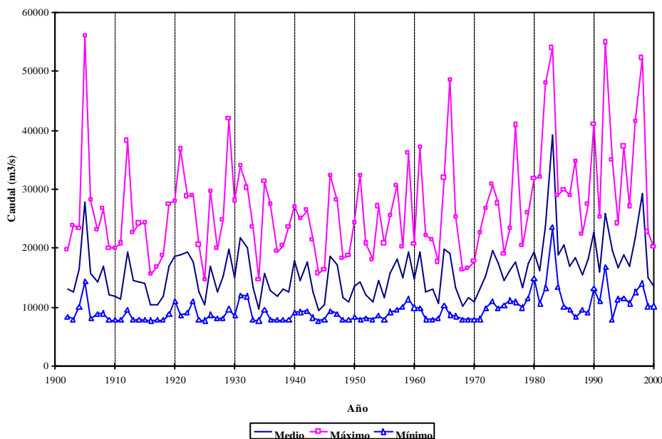
Figura 24 Máximos, mínimos y medios anuales de los caudales diarios del río Paraná en la sección Paraná-Santa Fe para el período 1902-2000
