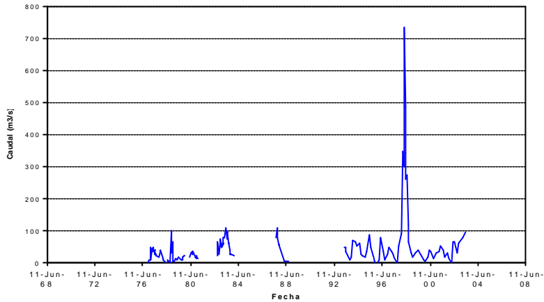
Figura 32 Serie de aforos del arroyo Batel
