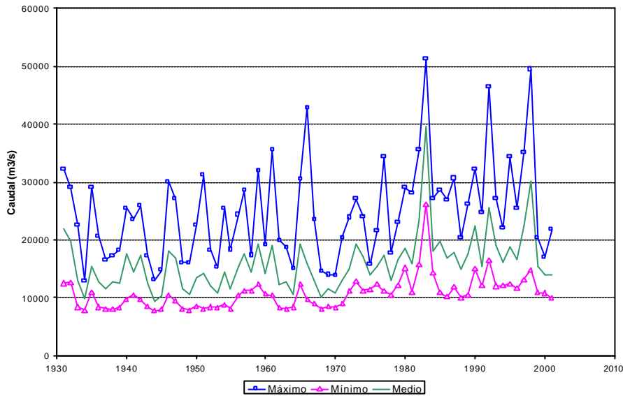
Figura 25 Máximos, mínimos y medios anuales de los caudales medios mensuales del río Paraná en la sección Paraná-Santa Fe para el período 1931-2001
