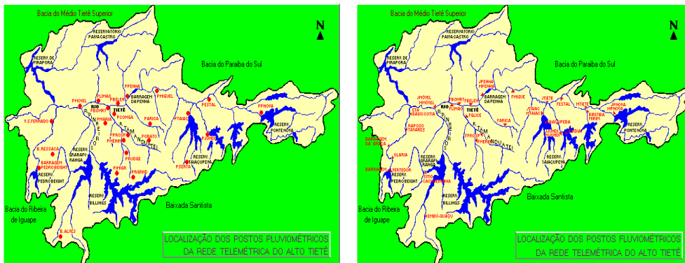
Figura 7. Red telemétrica pluviométrica y pluviométrica en la cuenca del Alto Tieté (Fuente: SAISP)
