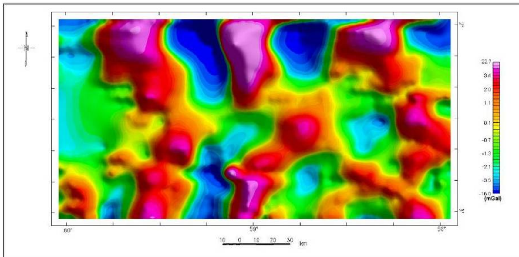
FIGURA 5.5 - Mapa de Anomalia Bouguer filtrado Passa Alta ( <100\text{ km} ). Foi aplicado um sombreamento artificial, com 45^\circ de azimute e 45^\circ de elevação da iluminação.
