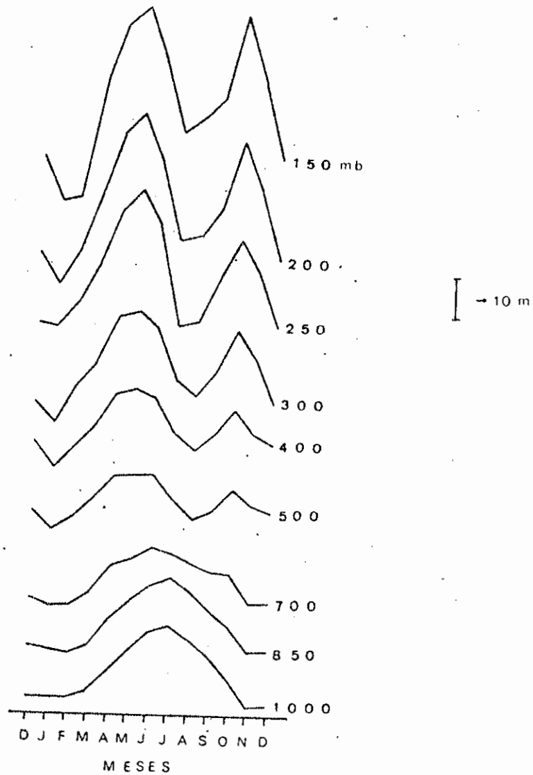
Fig. IV.2 - Desvios da altura geopotencial em relação à média anual (utilizando médias climatológicas), para cada nível (indicado do lado direito da figura) e o histograma de precipitação média mensal (1968 - 1976), para Belém.
