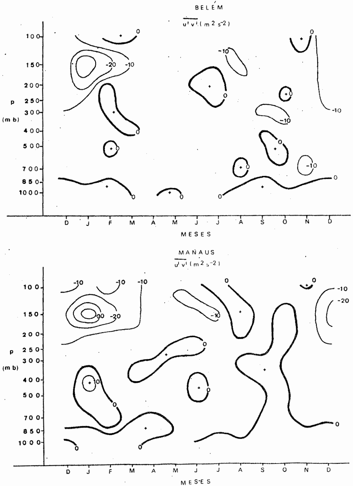
Fig. IV.17 - Seção "altura versus tempo" do transporte horizontal de quantidade de movimento feito pelos turbilhões transitentes, para Belém e Manaus.
