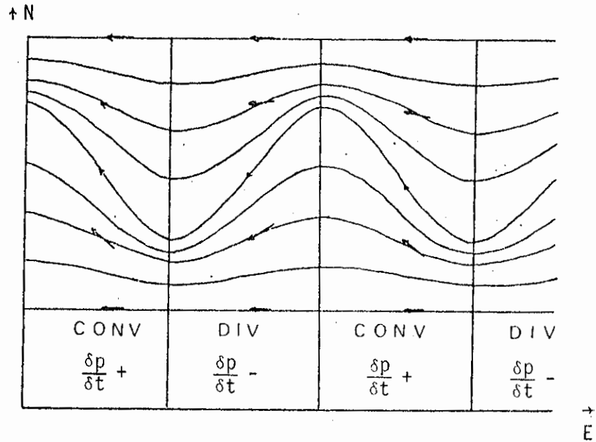
Fig. I.2 - Sistema de isóbaras divergentes e convergentes, para o hemisfério norte.
