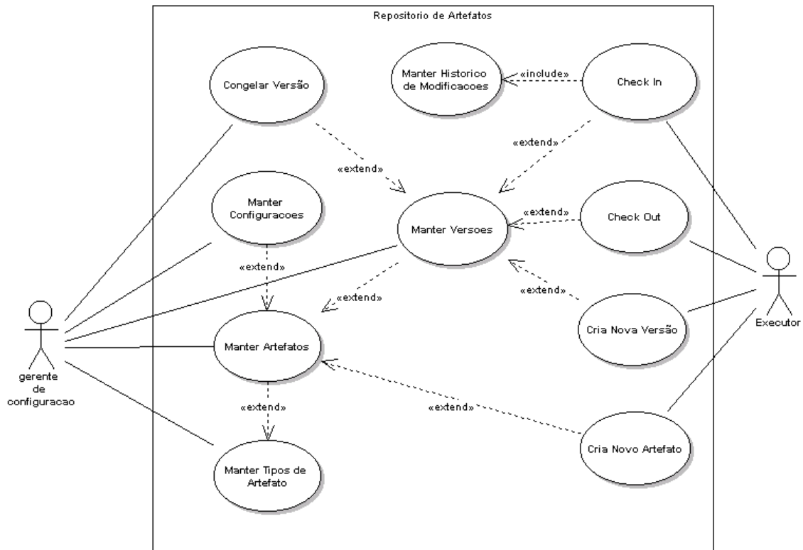
FIGURA 7.2.- Diagrama de Casos de Uso: Repositório de Artefatos.
