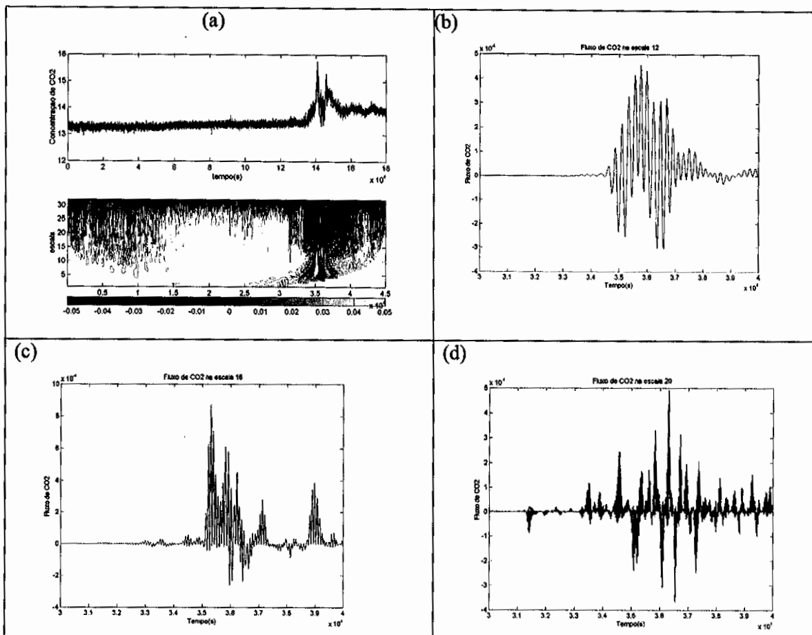
Figura 1. (a) Sinal bruto de CO 2 e análise de ondeleta em tempo-escala da parte real do coeficiente de CO 2 ; (b) projeção da ondeleta de Morlet na escala 12 do fluxo de CO 2 ; (c) projeção da ondeleta de Morlet na escala 16 do fluxo de CO 2 ; (d) projeção da ondeleta de Morlet na escala 20 do fluxo de CO 2 ;
