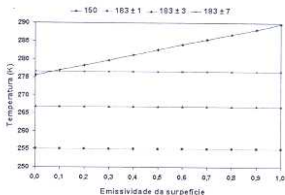
Figura 2 – Gráfico das Tb's(K) simuladas para cada canal em função da emissividade da superfície para céu claro e uma atmosfera tropical padrão. As curvas de TB_1 a TB_4 correspondem aos canais 150, 183 ± 1, 183 ± 3 e 183 ± 7 GHz, respectivamente.
