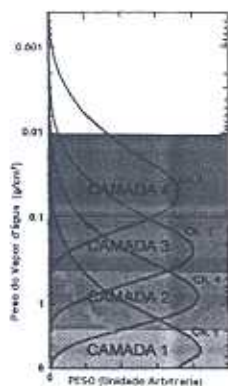
Figura 5 – Representação das camadas sobre as regiões de máximo das funções peso para cada canal do sensor HSB.
