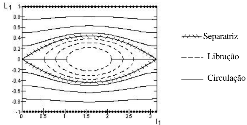
FIGURA 4.1 – Espaço de Fase (\bar{l}_1, L_1) para valores normalizados da Lua, para A < B < C , com F_A = 0,50031119 (ponto central com \bar{l}_1 = \pi/2 e L_1 = 0 ), F_B = 0,50025113 (separatriz, curva \text{---}\text{---}\text{---} ) e F_C = 0,5 ( L_1 = \pm L_2 , curva \text{---}\text{---}\text{---} )
