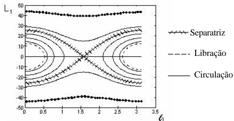
FIGURA 4.2 - Espaço de Fase (l_1, L_1) para satélite de pequeno porte, para B < A < C , com a separatriz definida pela curva \cdots .
