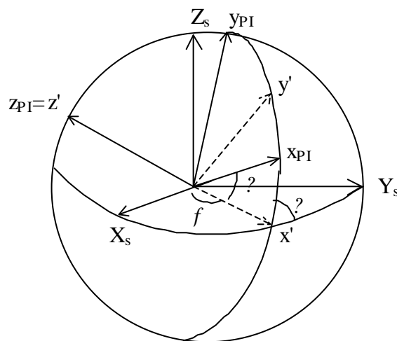
FIGURA 3.1 - Sistema principal ( Ox_{PI}y_{PI}z_{PI} ), Sistema do satélite ( Ox_s y_s z_s ) e os Ângulos de Euler ( f, ?, ? ), sistema intermediário ( Ox'y'z' )
