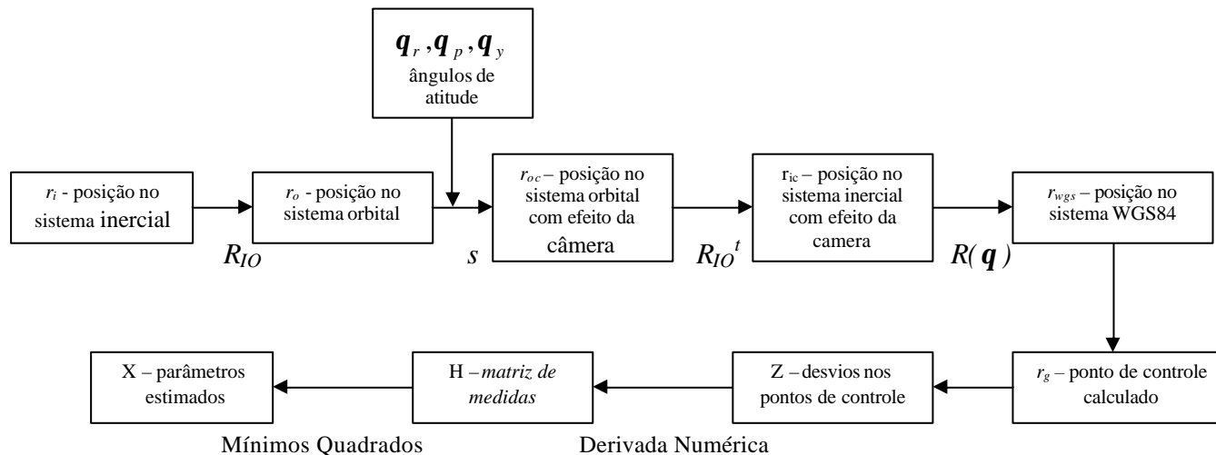
FIGURA 6.3 – Esquema para estimação dos desvios de atitude
