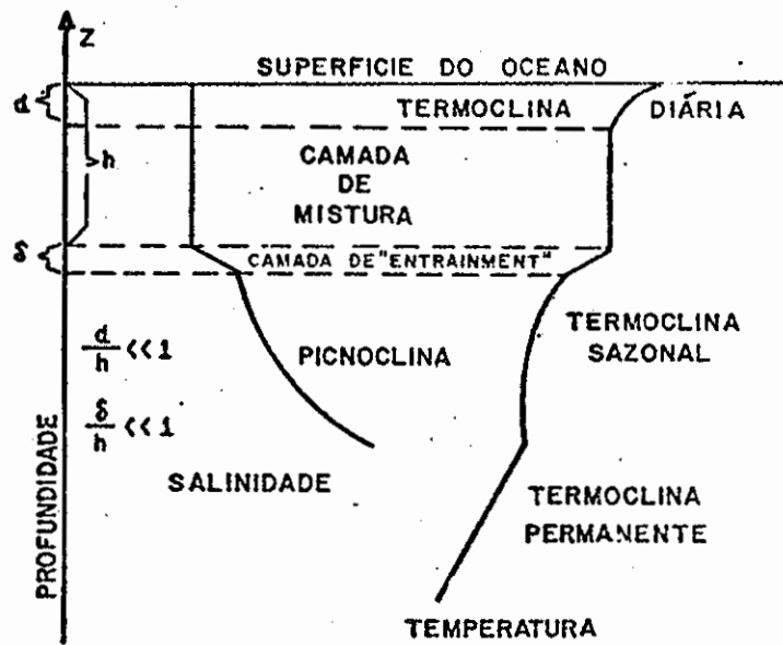
Fig. 3.2 - Representação esquemática da estrutura vertical do modelo de c.m.: d, espessura da região dominada pelas ondas; h, espessura da c.m.; \delta , espessura da c.e..
