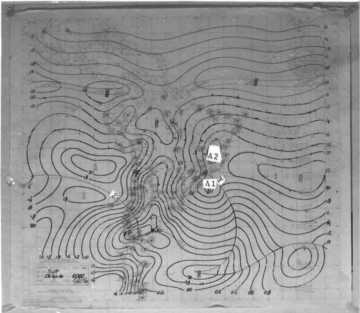
Fig. 4.9 - Cartas sinóticas de superfície oriundas do IAE para o período de 28 a 31 de julho de 1980.
