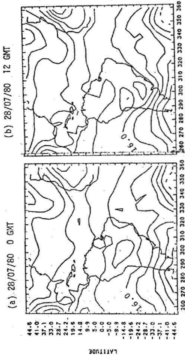
Fig. 4.5 - Temperatura em 85 kPa para o período de 28 a 31 de julho de 1980. Contorno de - 4 a 40 e intervalo de 4 ( ^{\circ} C).
