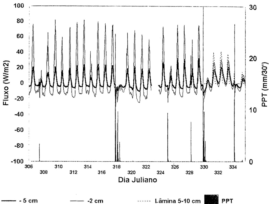
Fig. 1 – Precipitação pluviométrica e fluxos de calor no solo (FCS) e na lâmina de água (FCL) em Passo do Lontra, MS, no mês de novembro de 2000
