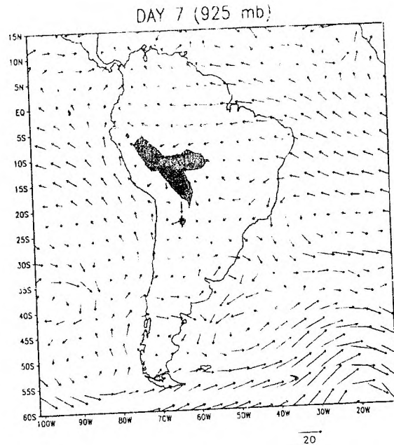
Figura 2 - Dispersão de mercúrio na atmosfera, no sétimo dia após início, em 20/08/96, de emissão constante por cinco dias, a partir de uma fonte localizada em Alta Floresta
