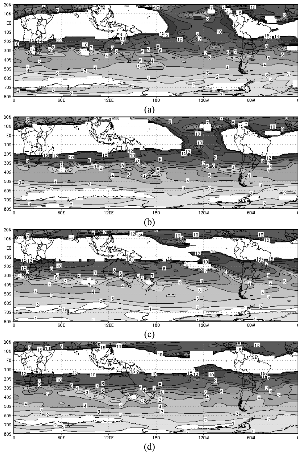
Figura 6.4 - k_s para o nível de 300 hPa para casos: a) secos e b) úmidos de verão, c) secos e d) úmidos de outono, e) secos e f) úmidos de inverno, g) secos e h) úmidos de primavera. Regiões com k_s maior do que 15 não são sombreadas. Continua ...
