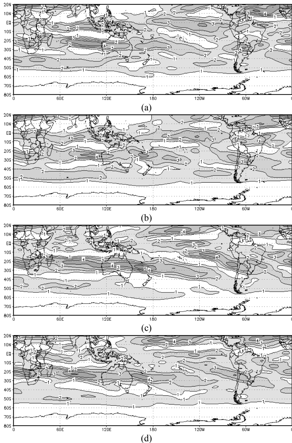
Figura 6.3 - Gradiente meridional da vorticidade absoluta em coordenadas Mercator para casos: (a) secos e (b) úmidos de verão, (c) secos e (d) úmidos de outono, (e) secos e (f) úmidos de inverno, (g) secos e (h) úmidos de primavera. Valores acima de 1 \cdot 10^{-11} \text{ s}^{-1} \cdot \text{m}^{-1} são sombreados. Continua...
