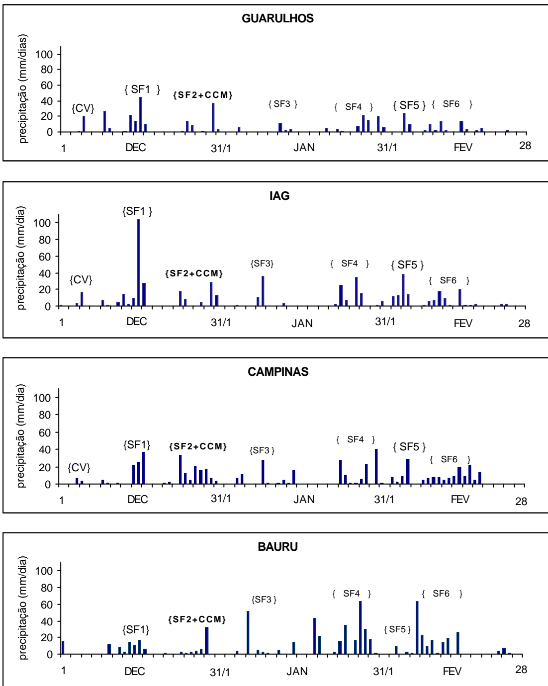
FIGURA 5.6 - Distribuição da precipitação nas estações de GR, IAG, KP, BR, PP e RP localizadas no estado de São Paulo durante o verão 2000 – 2001.
