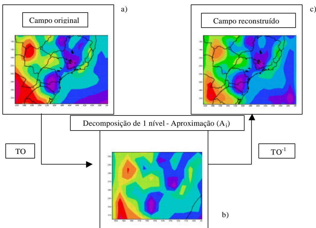
FIGURA 3.5 – Decomposição num nível do campo de temperatura em 1000 hPa, derivado do modelo T126 do dia 18 de janeiro de 2001: campo de temperatura original (a), campo decomposto num nível (b) e campo reconstruído (c).
