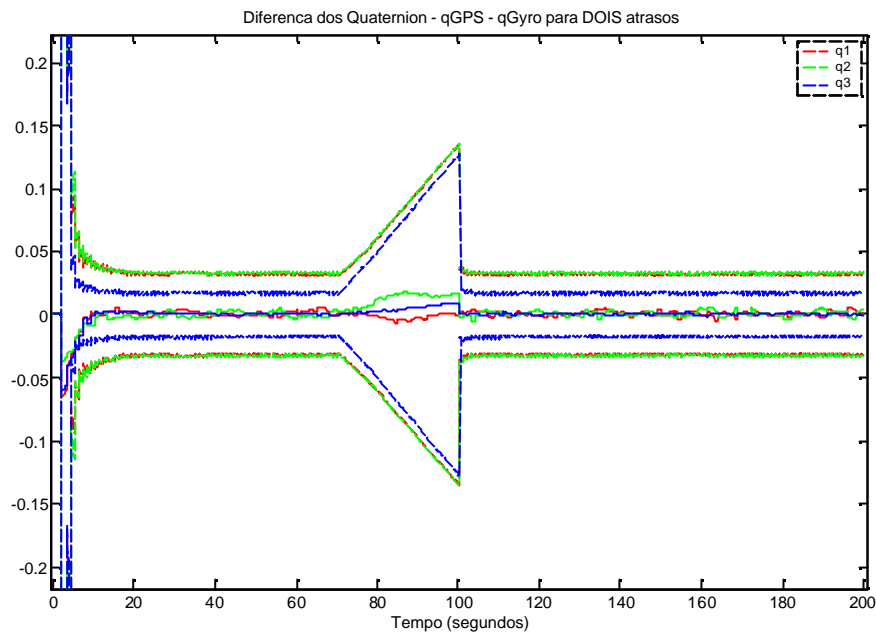
FIGURA 4.59 – Diferença dos quatérnio – qGPS – qGiro para dois atrasos, e faixa de incerteza (2 sigmas).
